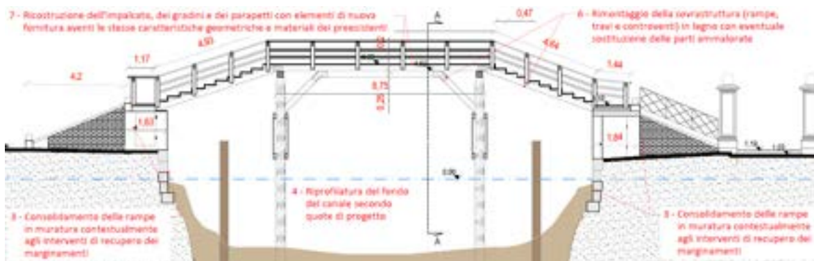
TRAFFICO 3.1.4.1 - Sezione Spingola d'Intervento 3.1.4.1 (Stato di fatto) - Progetto Definitivo - Sezione TRAF 3.1.4.1
